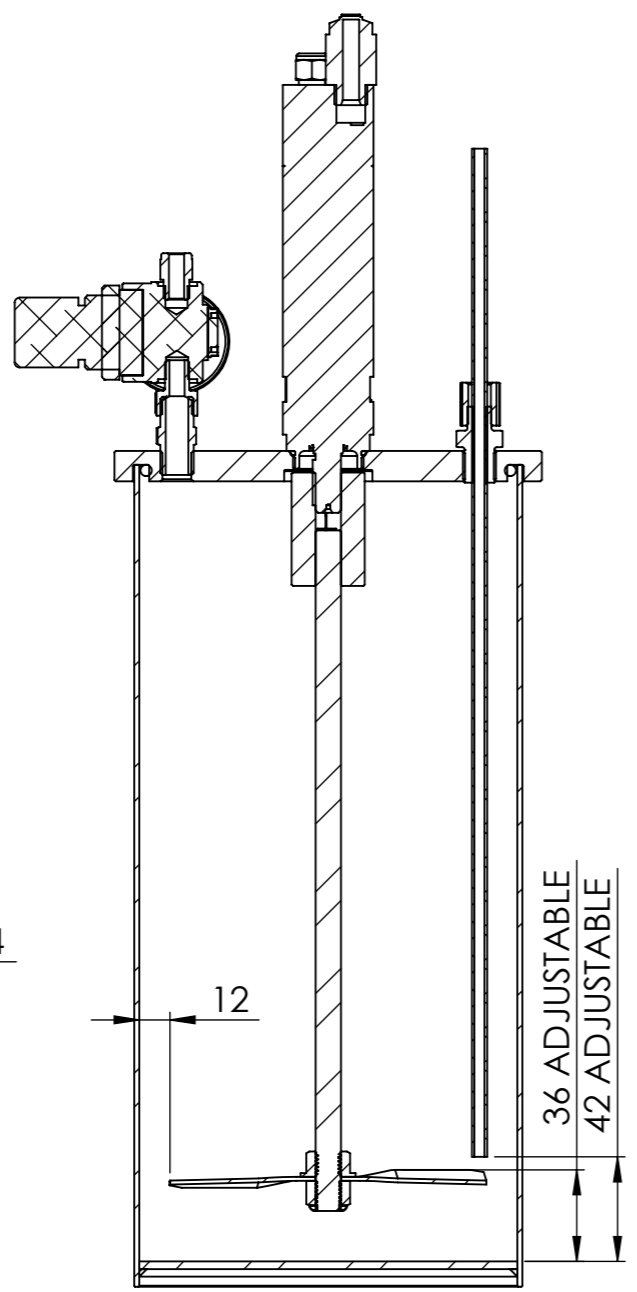
COUPE A-A
